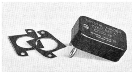
TYPE 560-A Crystal Holder
