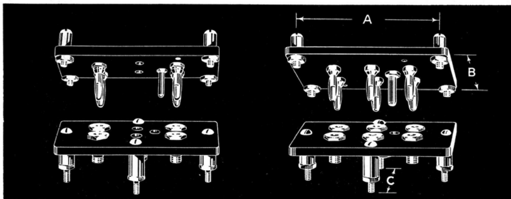
TYPE 274-EP TYPE 274-EJ
